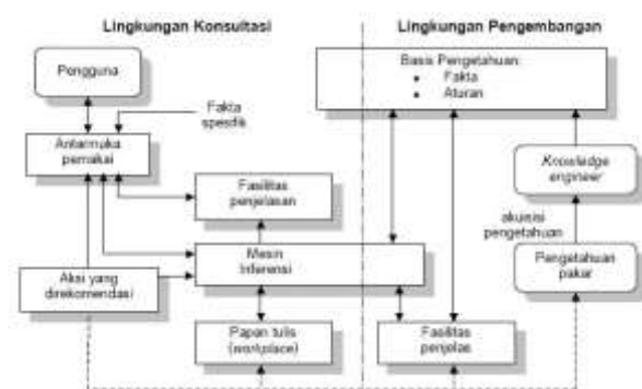
Gambar 1. Arsitektur dari Sistem Pakar
