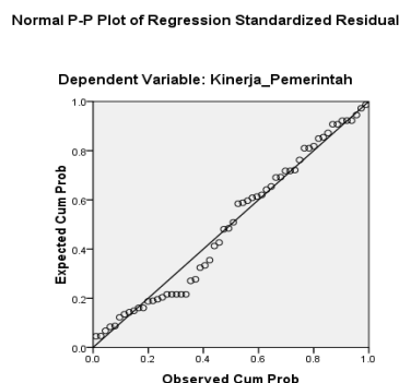
Gambar 1. Uji Normalitas
